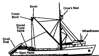
Purse Seiner
